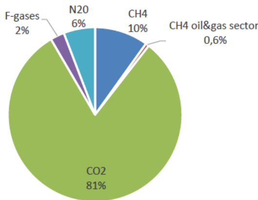
Figura 3.8: Emissioni di gas serra in EU (2019)
